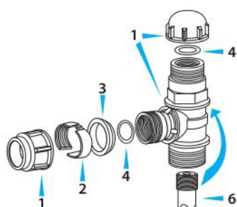
for PE Pipes Connection
